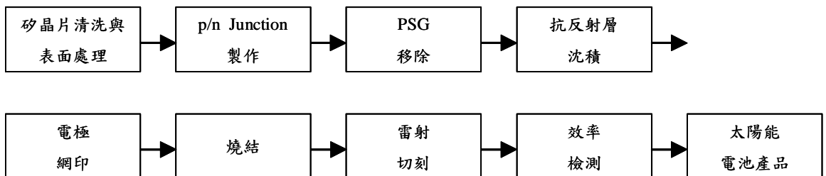
圖7、結晶矽太陽能電池製造流程
